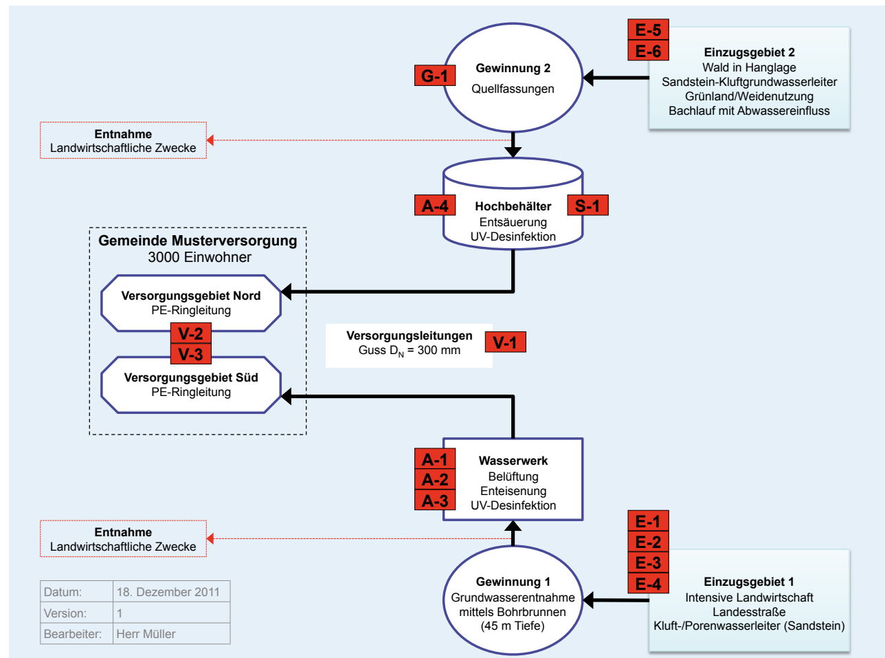
Abbildung 9: Musterversorgung – Fließschema mit identifizierten Gefährdungen (nach Tabelle 3)
