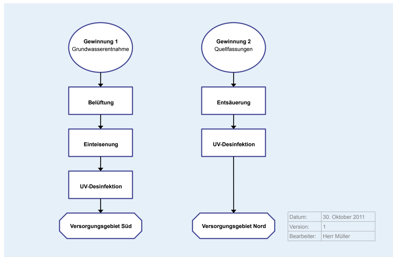
Abbildung 7: Musterversorgung – Aufbereitungsschema
