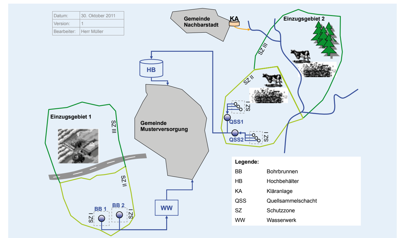
Abbildung 5: Musterversorgung – Übersichtsplan
