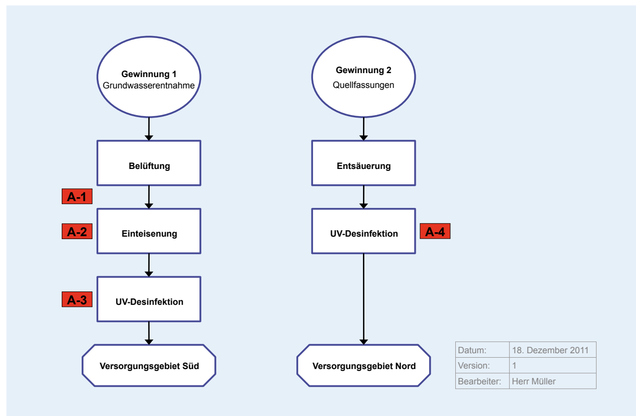
Abbildung 10: Musterversorgung – Aufbereitungsschema mit identifizierten Gefährdungen (nach Tabelle 3)
