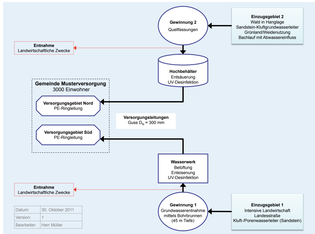
Abbildung 6: Musterversorgung – Fließschema
